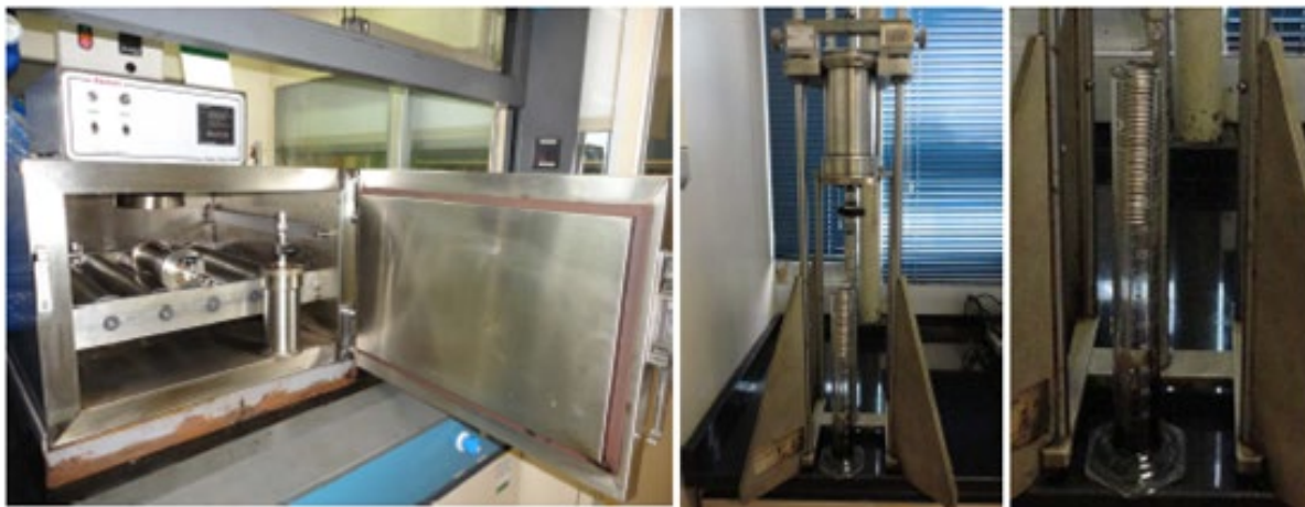
Figura 2 – Exemplos dos equipamentos: (1) estufa roller oven FANN modelo 705ES, (2) suporte para acomodar a célula de pressão e (3) detalhe da acomodação da haste de tubo espiral dentro da proveta.
